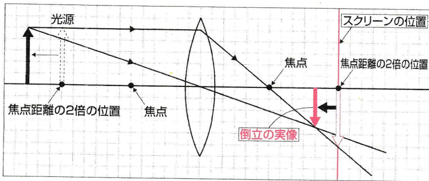
② 焦点距離の2倍より遠ざけた場合
